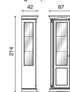
L. 67 P. 42 H. 214
