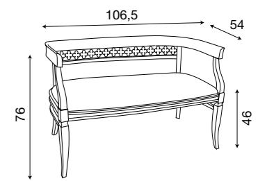
L. 106,5 P. 54 H. 76 seduta H. 46
